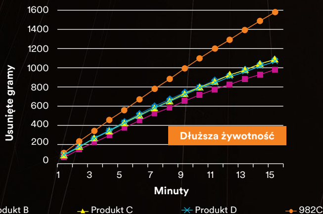
Wynik szlifowania
